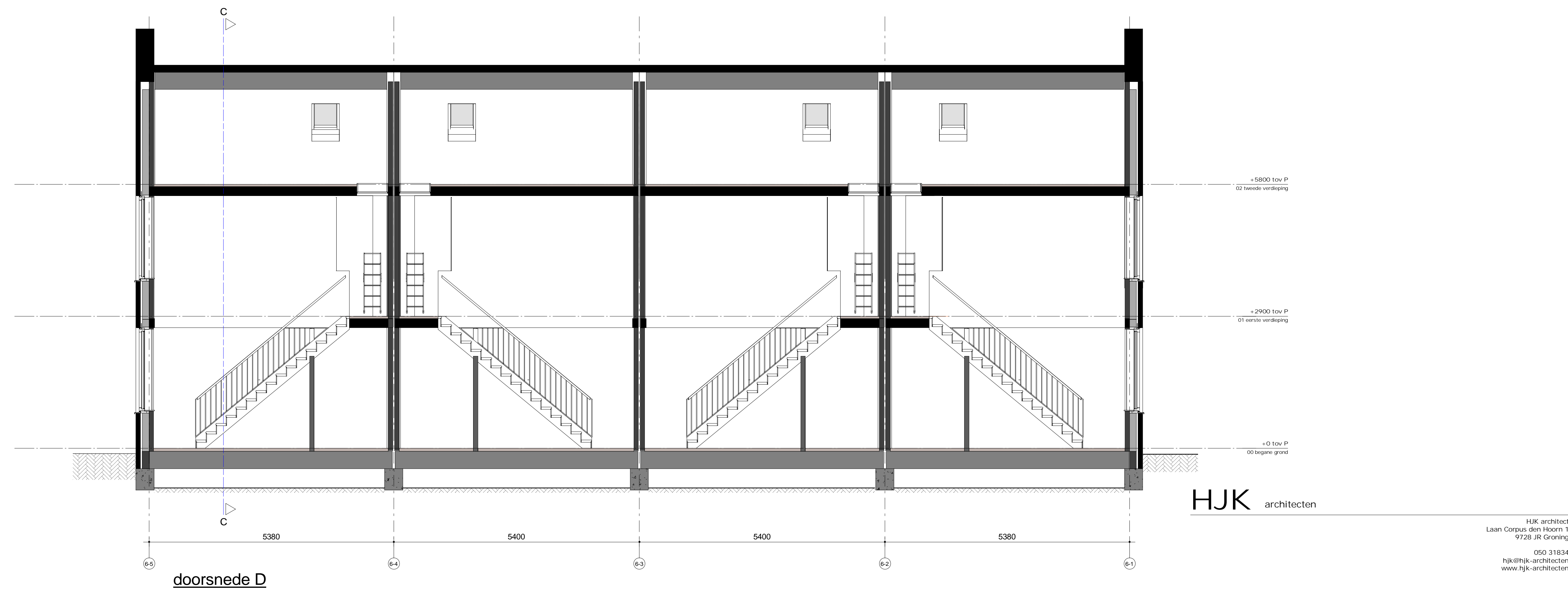
doorsnede D
