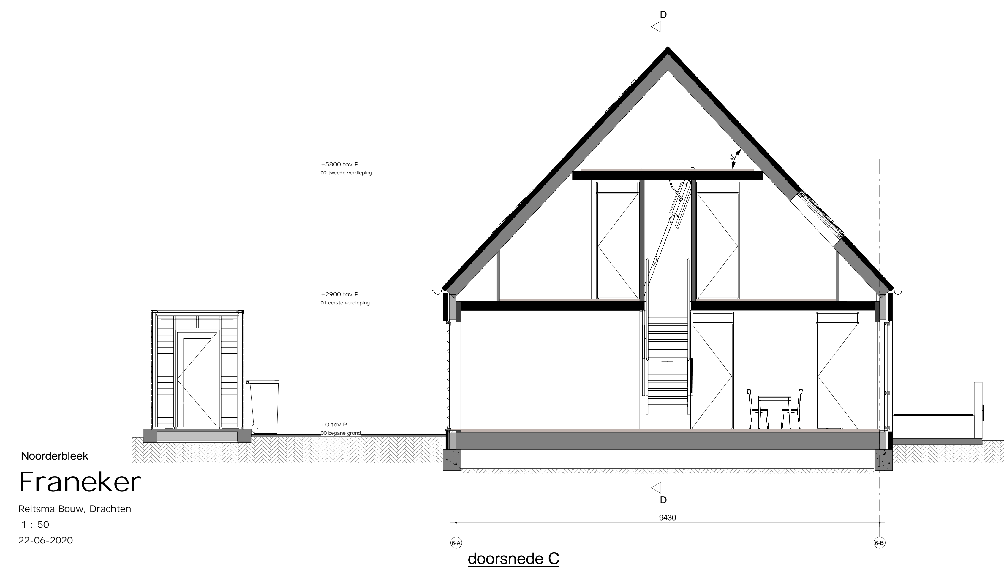
doorsnede C
